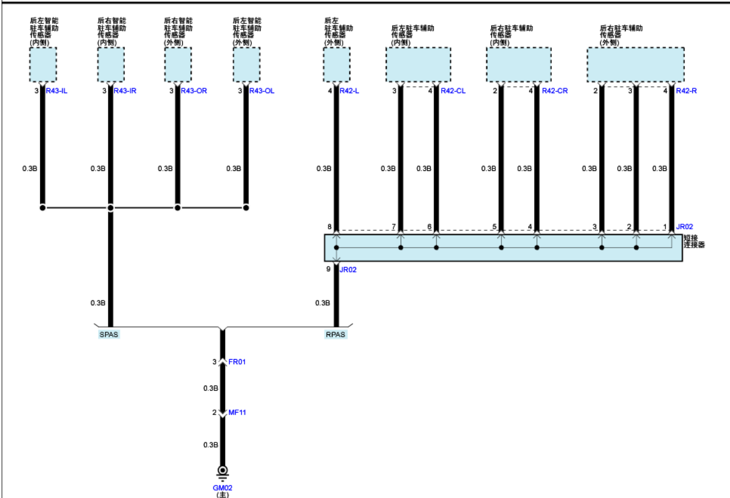
搭铁分布(4)
